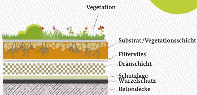
Aufbau eines Gründaches als Kaldach
