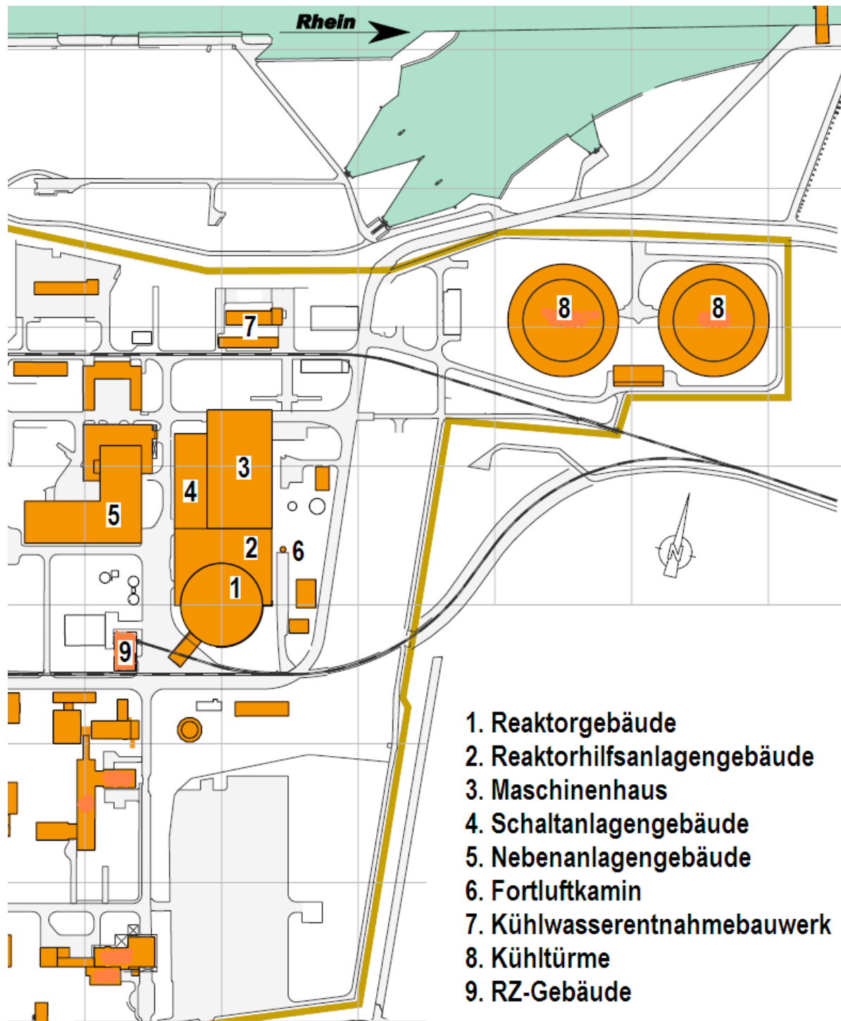
Abbildung 8: Lageplan KWB-A
