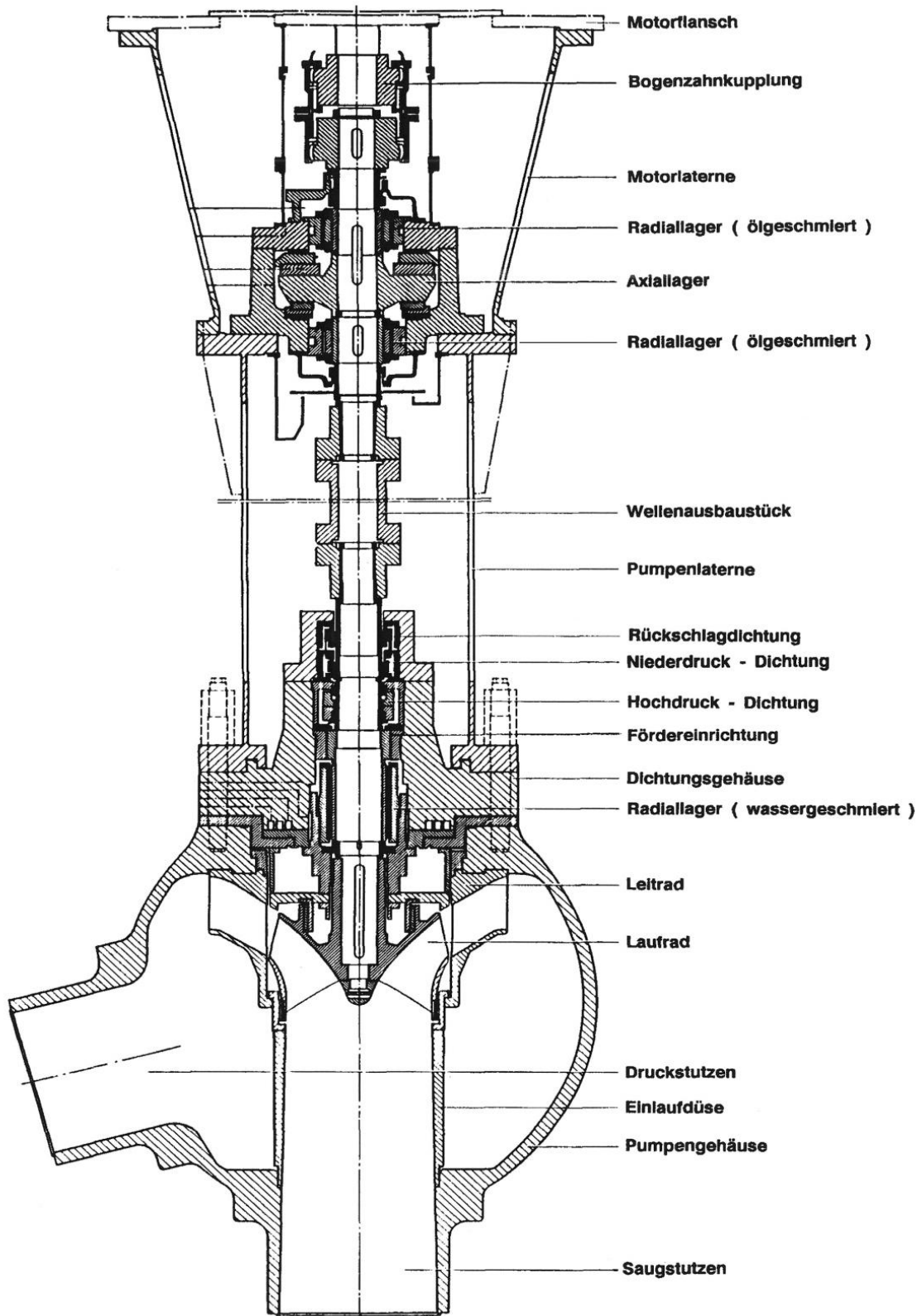
Abbildung 14: Hauptkühlmittelpumpe KWB-A
