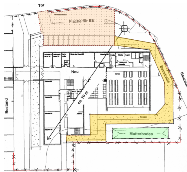
Baustelleinrichtung planen. © Ingenieurbüro Detlef Bartsch, Aachen (verändert)
